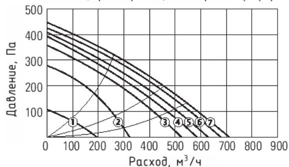
ПРИТОК, фильтр EU7, водяной калорифер
